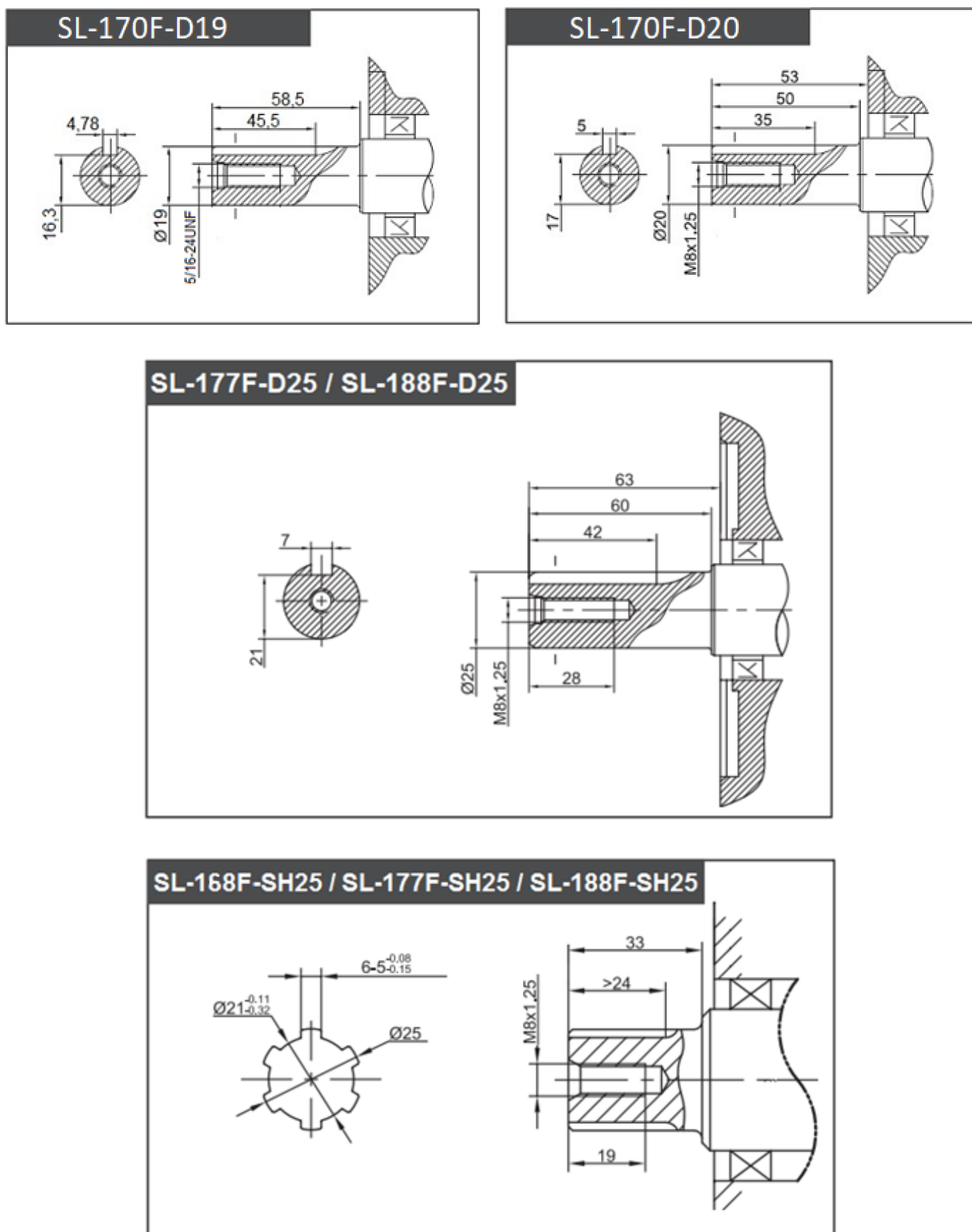
Рис. 2 – Типы валов
