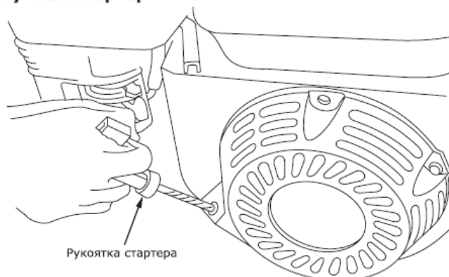
Рис. 12 – Ручной стартер
